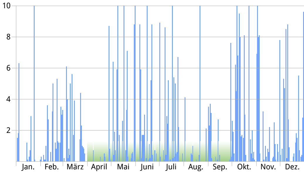
Abbildung 4: Niederschläge in mm/Liter pro Quadratmeter im Jahr 2009 (Quelle: Berechnungen aus Daten des DWD), Gießtage als Markierungen (grün)
