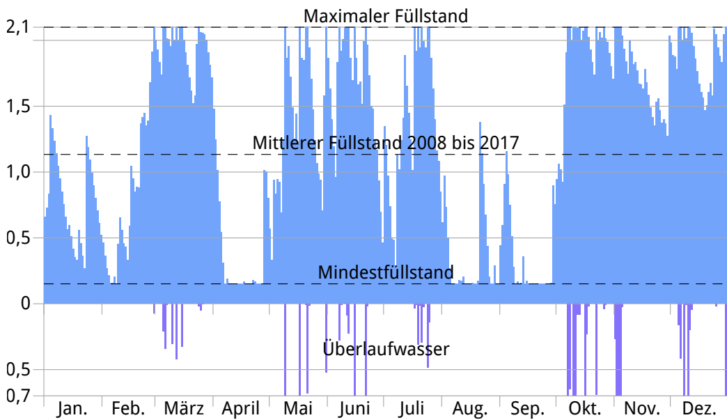
Abbildung 5: Zisternenfüllstände und Überlaufwasser in Kubikmeter/1.000 Liter im Jahr 2009
