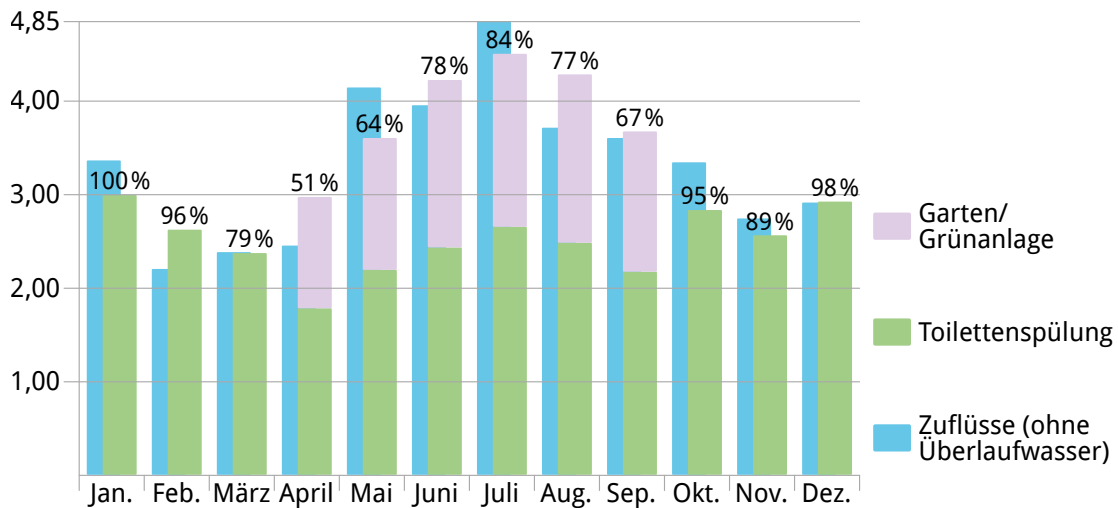
Abbildung 6: Durchschnittliche Regenwasserzuflüsse und -verbräuche in Kubikmeter/1.000 Liter mit Gesamtdeckungsgraden nach Kalendermonaten
